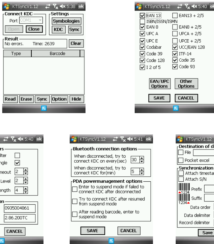
図 31- Mobile pKTSync
