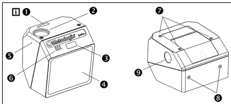
図1a. スキャナー構成部品
