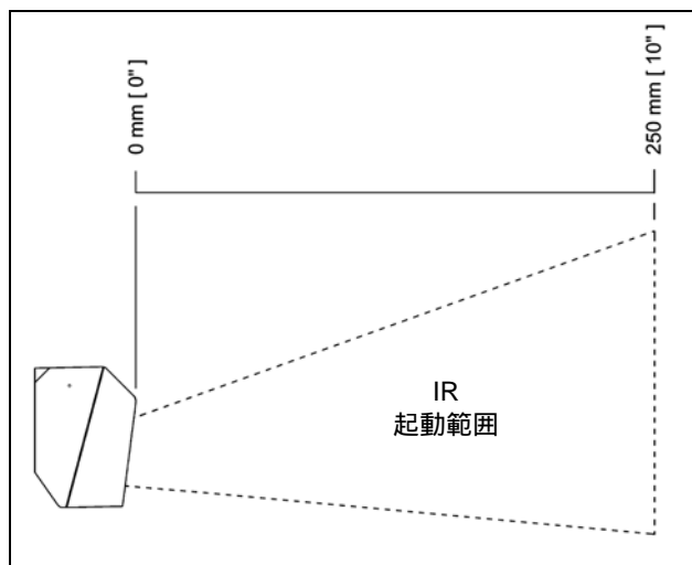
図 13. IR 標準起動範囲
