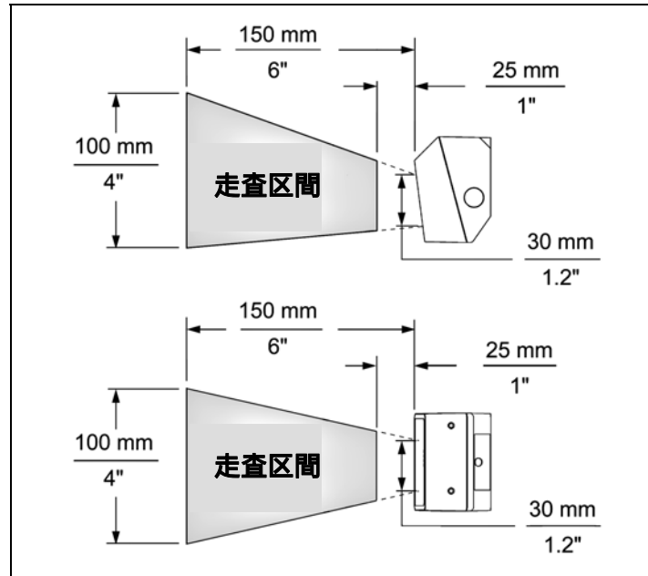
図 10. 低減フィールド深度
