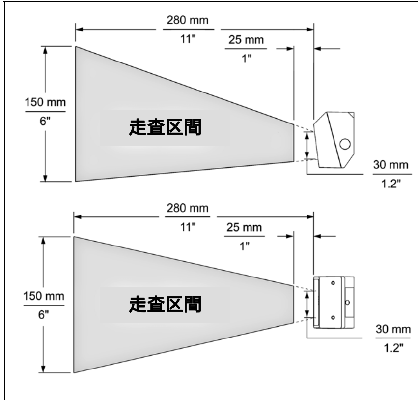
図9. 標準のフィールド深度
