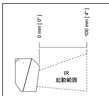
図 14. Reduced IR 起動範囲
